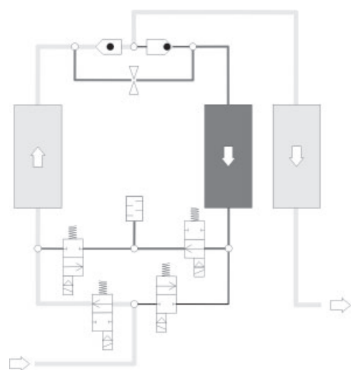
Régénération dans la chambre à agent dessiccant de droite
