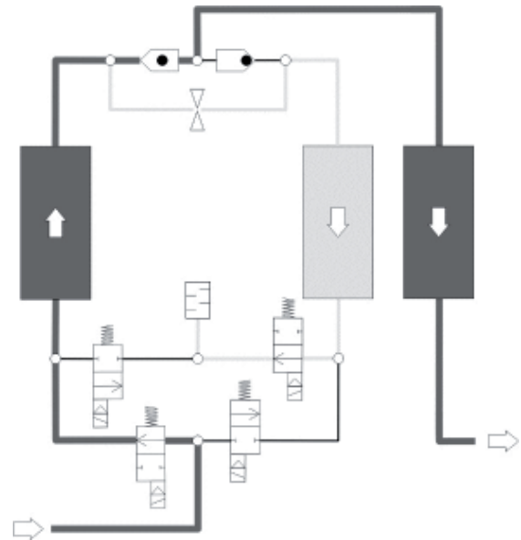
Adsorption dans la chambre à agent dessiccant de gauche
