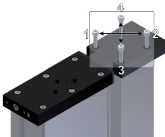
Fixer la plaque supérieure
